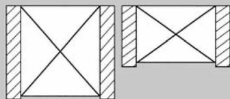
Korpus-Einzelbauweise mit Tiefenversatz
