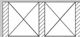
Korpus-Reihungsfähig ohne Tiefenversatz
